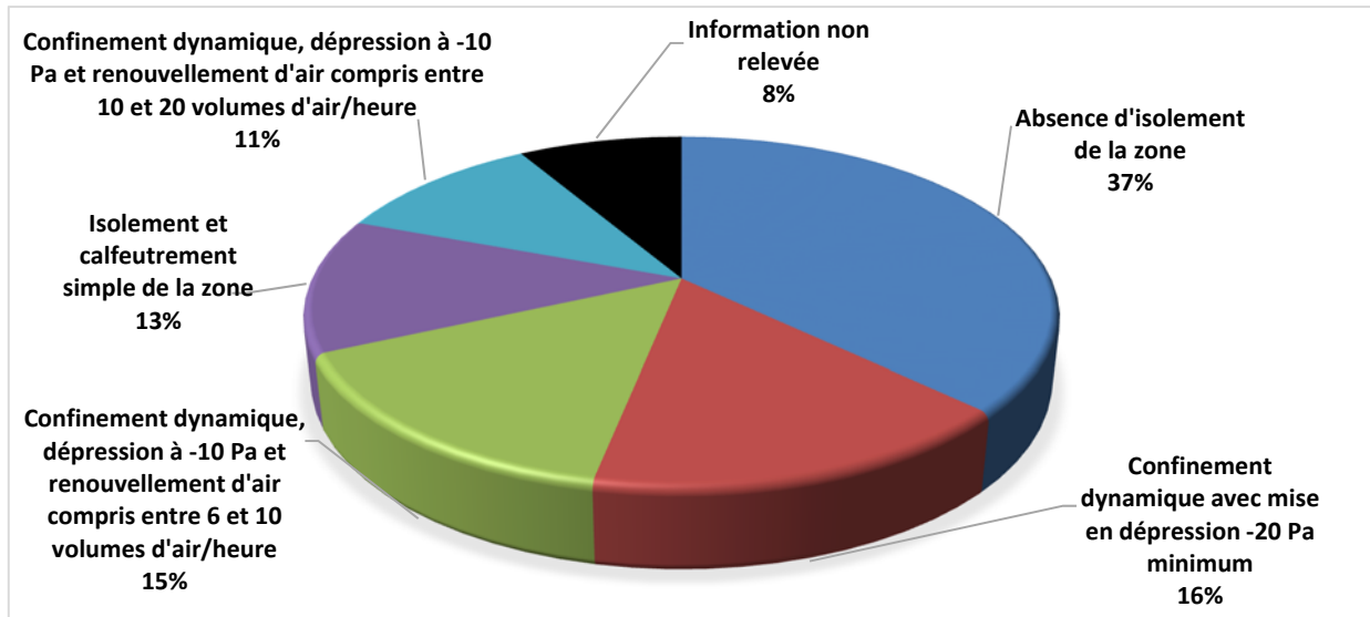
Figure 4 : Répartition du nombre de mesures par type de confinement
