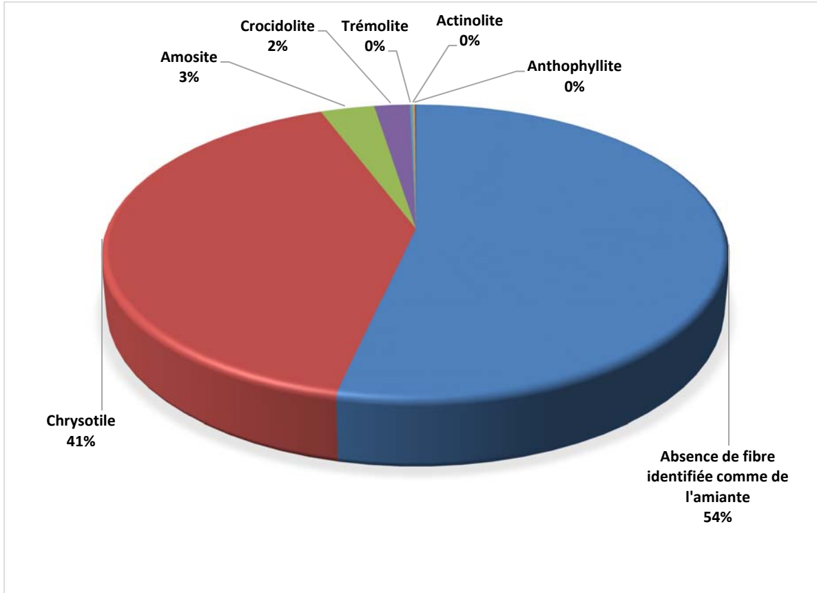
Figure 10 : Répartition du nombre de mesures par nature de fibre
