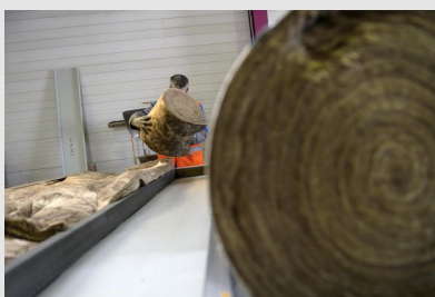
Manipulation de laines minérales d'isolation sous forme de rouleaux
