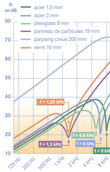
Indice d'affaiblissement et fréquence critique de quelques parois usuelles en fonction de la fréquence
