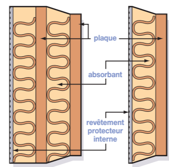
Paroi double, paroi simple
