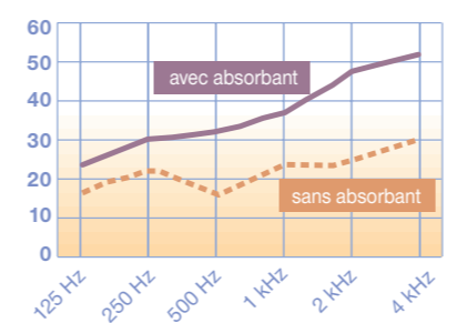
Exemple d'isolement d'un encoffrement avec et sans laine minérale en fonction de la fréquence
