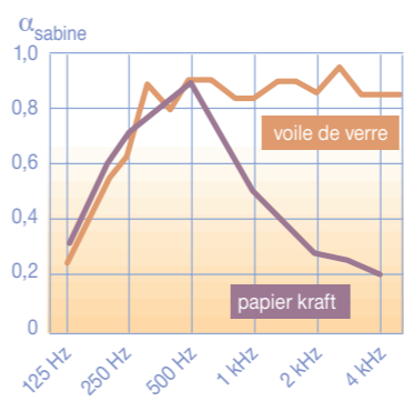
Influence d'un revêtement protecteur en fonction de la fréquence
