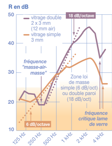
Indice d'affaiblissement d'un simple vitrage et d'un double vitrage en fonction de la fréquence
